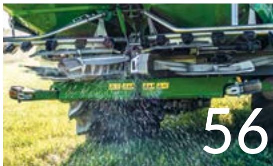
Rozsiew graniczny z Amazone BorderTS
